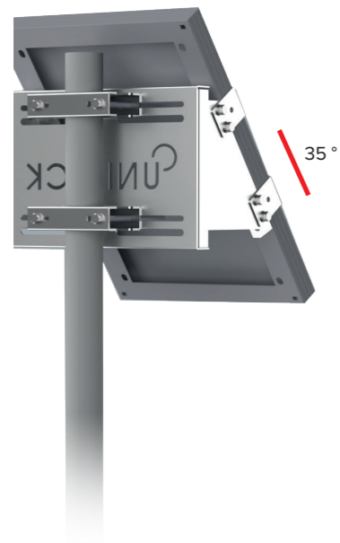
UNIFIX 5SF Pour Unisun 5.12 M Orientation portrait Tête et milieu de mât Brides de fixation en option Ref 2693
