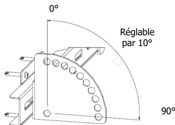
Performance électrique en fonction de l'inclinaison et de l'orientation panneau
